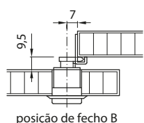
posição de fecho B
