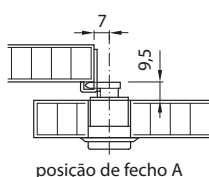
posição de fecho A
