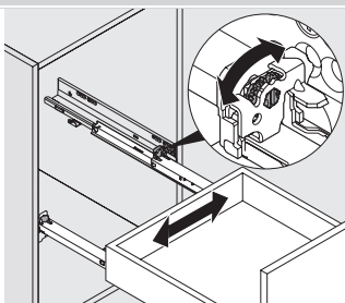
Regulagem lateral Compensação com corredeira direita posterior
