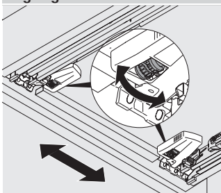
Regulagem lateral Bilateralmente com acoplamento \pm 1.5 mm
