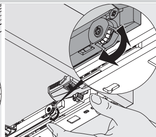
Regulagem de profundidade Com TIP-ON - 1/+ 2 mm
