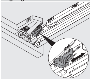
Regulagem da altura + 3 \text{ mm}
