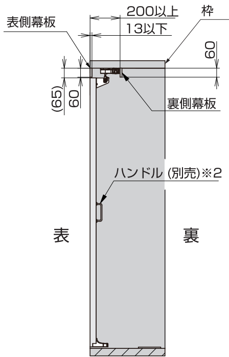
上カーブレール①取付詳細図
