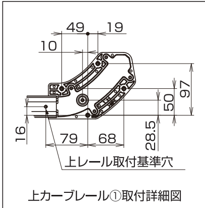
側板加工詳細図
