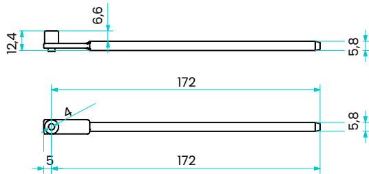
HASTE CURTA (2ADSR042)
