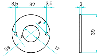
ESPAÇADOR DA FECHADURA (2ADSP039017002)
